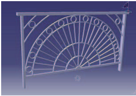
Conception (Calculs de structure et Design) d'une rembarde de pont à Vierzon
